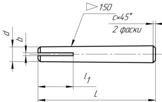
Рис. 2. Таблица параметров и изображение штифта с именами переменных
