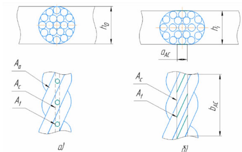
Рис. 3 Схема формирования контурной и фактической площади контакта в системе «канат – поверхность»
