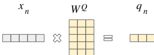
Рис. 1. Получение вектора запросов
