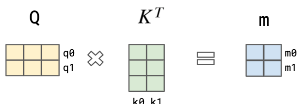
Рис. 4. Вычисление значимости
