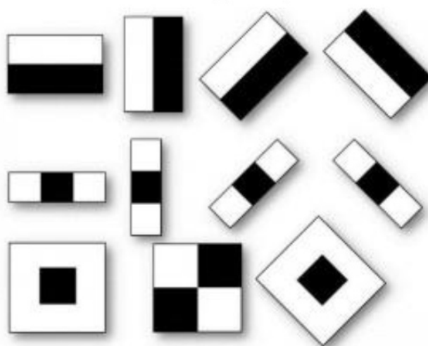
Рис 3. Примитивы Хаара
