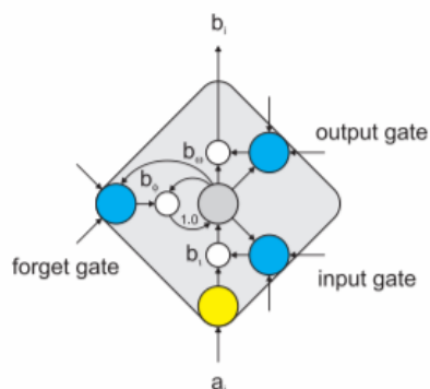
Рис. 3.LSTM: ячейка памяти
