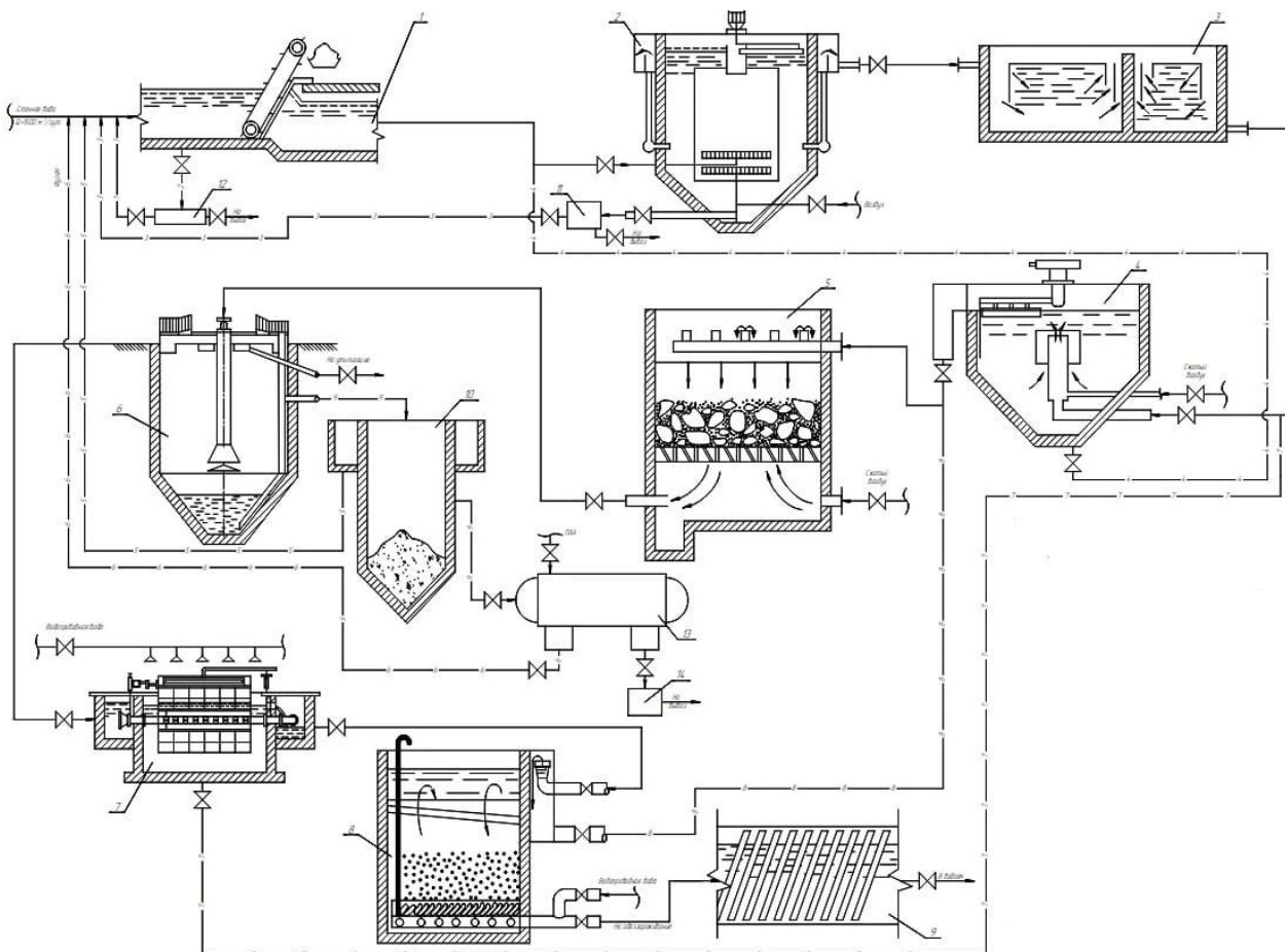
Рис.1. Технологическая схема очистки сточных вод маслоэкстракционного завода: 1 - механическая решетка; 2 - аэрируемая жироловушка, 3 - прямоугольный усреднитель; 4 - напорный флотатор, 5- капельный биофильтр; 6- вертикальный отстойник; 7- барабанная сетка; 8 - скорый фильтр с загрузкой; 9 - УФ-установка; 10- осадкоуплотнитель; 11- сборник после жироловушки 12- сборник осадка после механической решетки ;13- центрифуга ; 14- сборник после центрифуги
