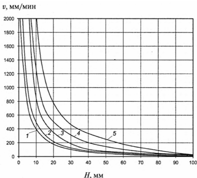
Рис. 1. Зависимость средних значений скоростей резания некоторых метриалов от их толщины:
