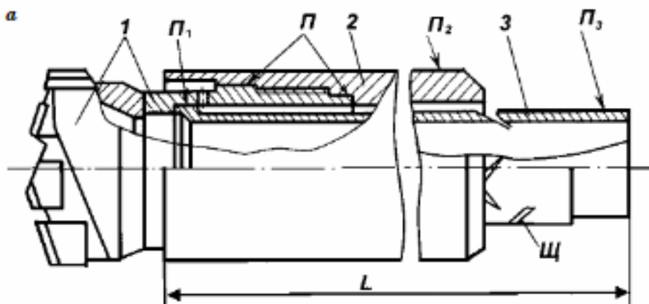
Рис 3. Эжекторное сверло
